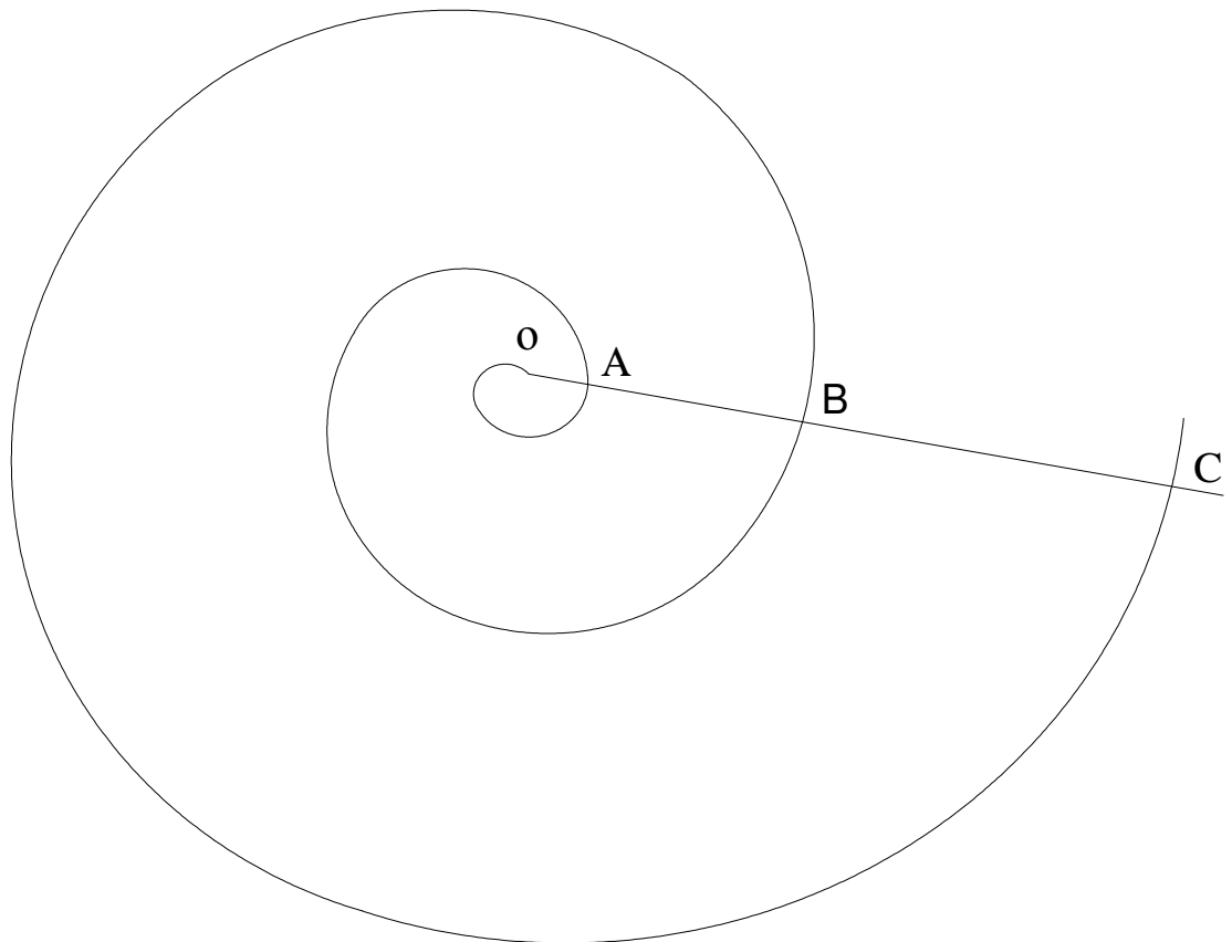
Рис.4.5. Логарифмічна спіраль
