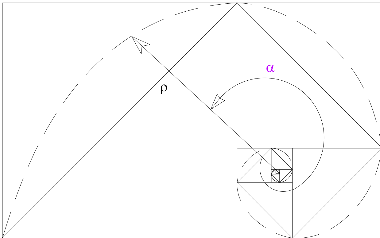
Рис.2 Спіраль Фібоначчі
