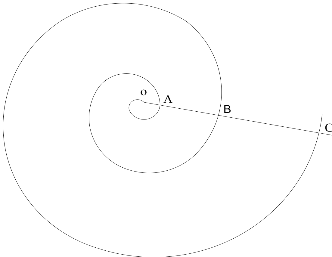
Рис.3. Логарифмічна спіраль
